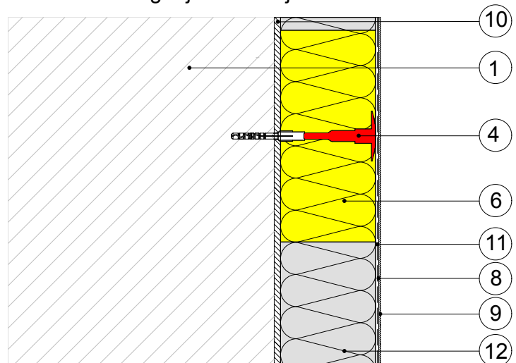
b) Baumit SchraubDübel Speed s pasom negorljive izolacije
