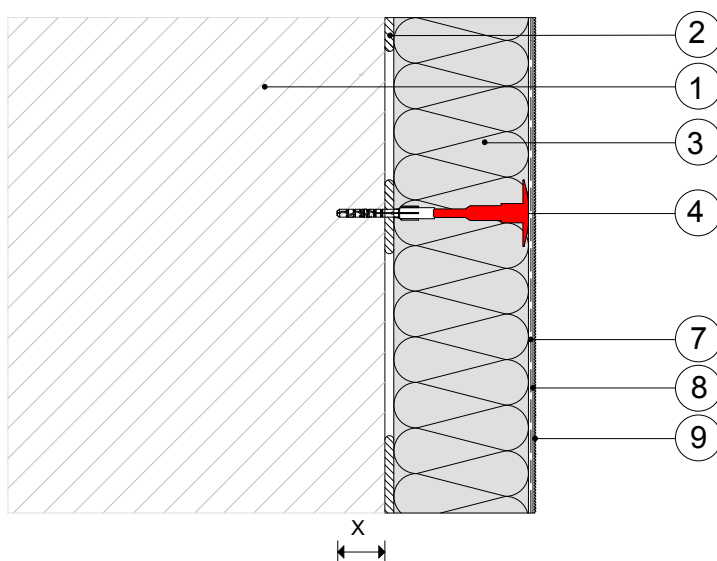
c) Baumit SchraubDübel Speed poravnan s površino
