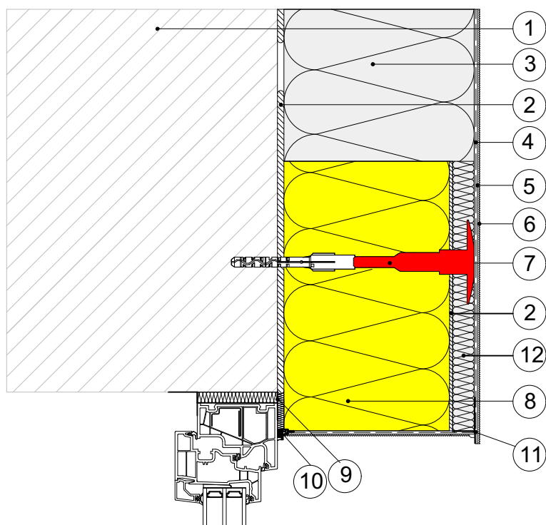
b) Izvedba pri oknih poravnanih z zidom
